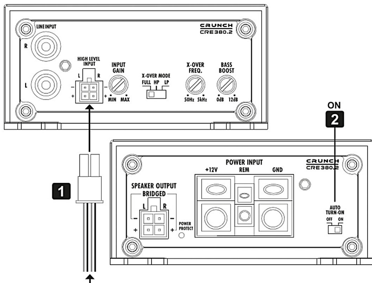
Rys. 6 — Wejścia wysokopoziomowe i automatyczne włączanie. Sygnał z kabli głośnikowych radia; przełącznik AUTO TURN-ON w pozycji ON.
