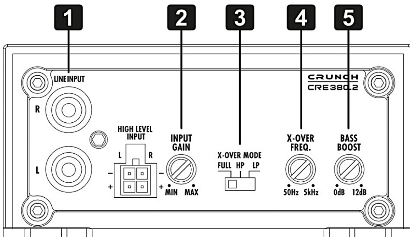
Rys. 1 — Przyłącza i elementy sterowania
