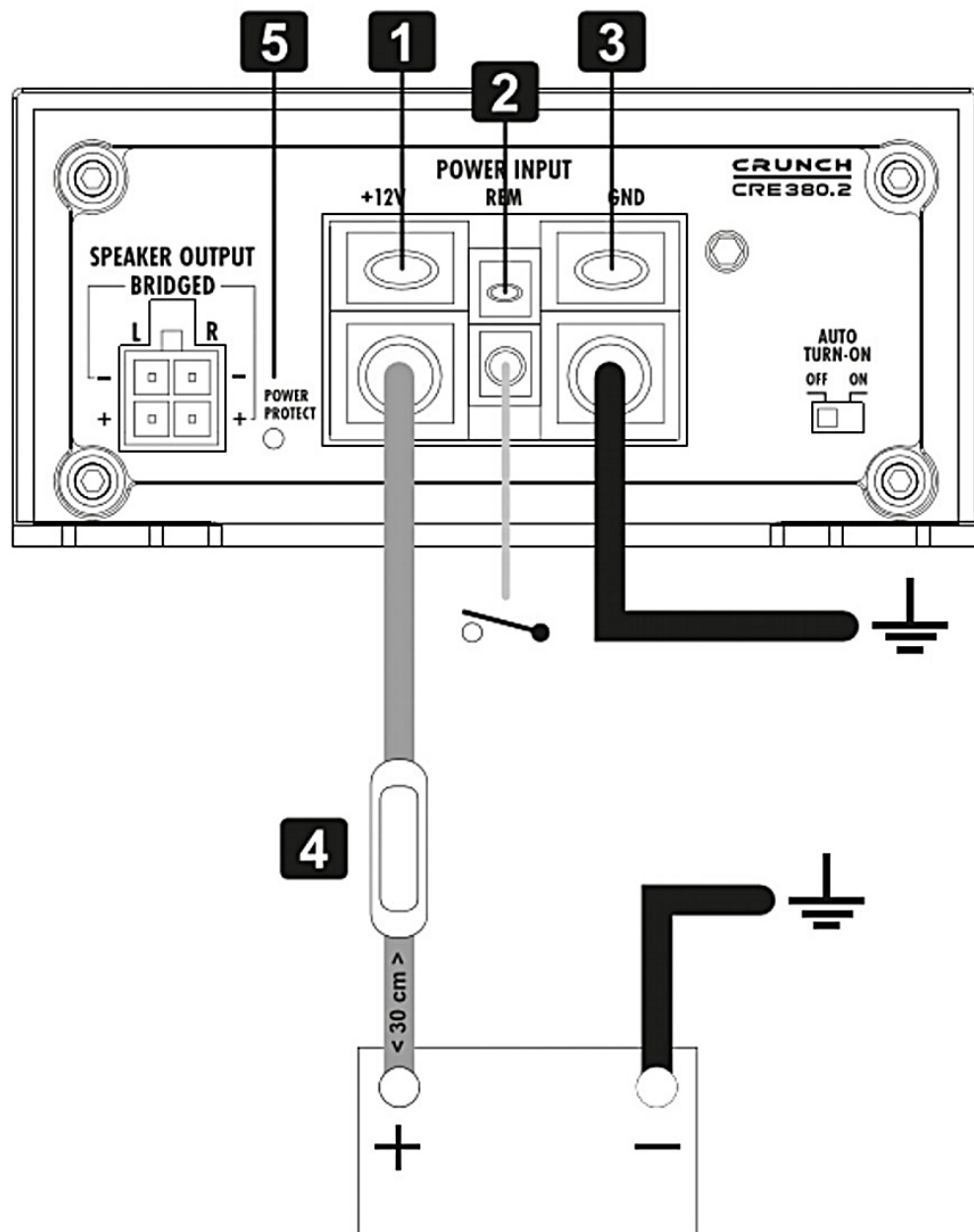
Rys. 2 — Podłączenie zasilania (1: +12V • 2: REM • 3: GND/masa • 4: zewnętrzny bezpiecznik kabla • 5: dioda statusu)
