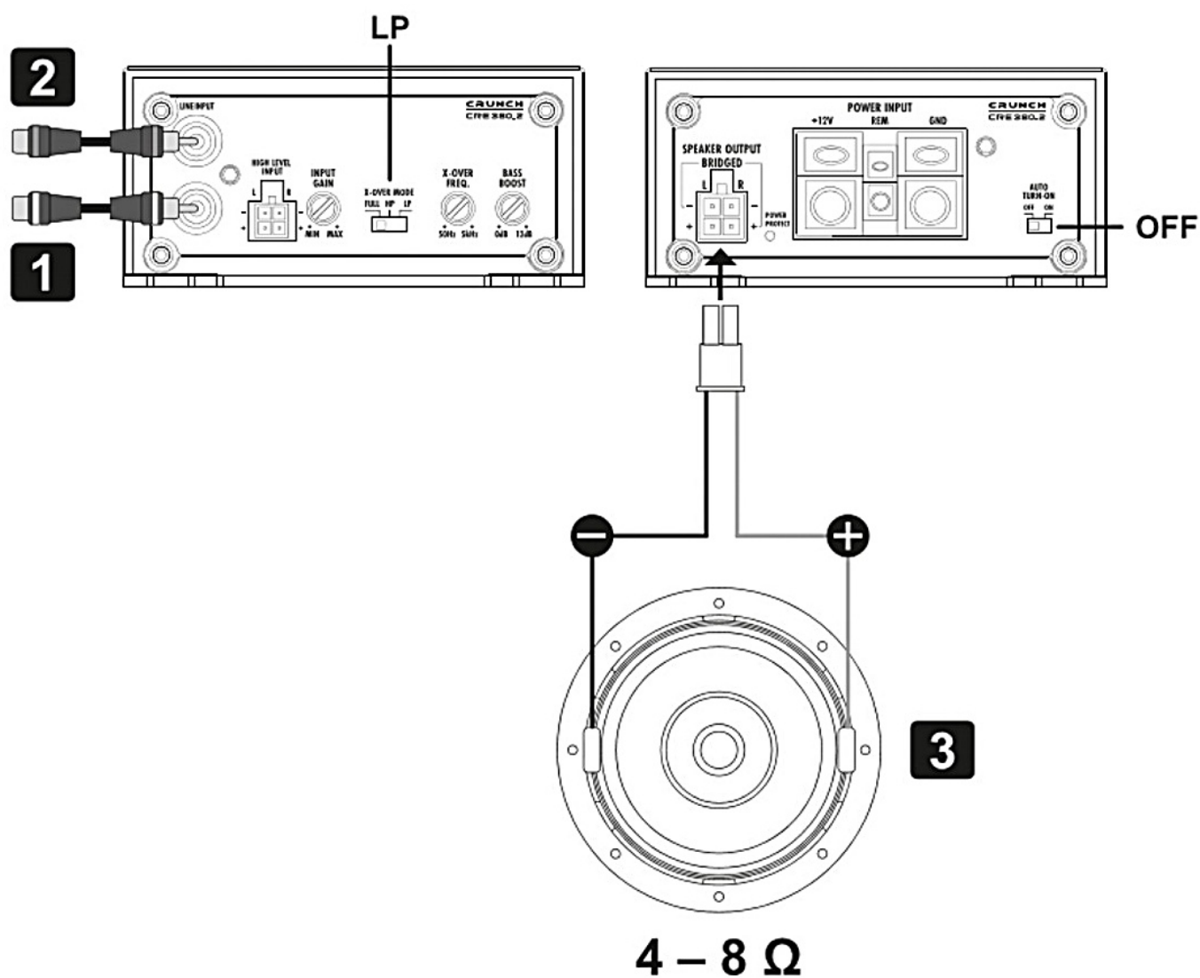
Rys. 4 — Praca mono. Subwoofer podłączony do wyjścia mostkowanego; impedancja minimalna 4 Ω.
