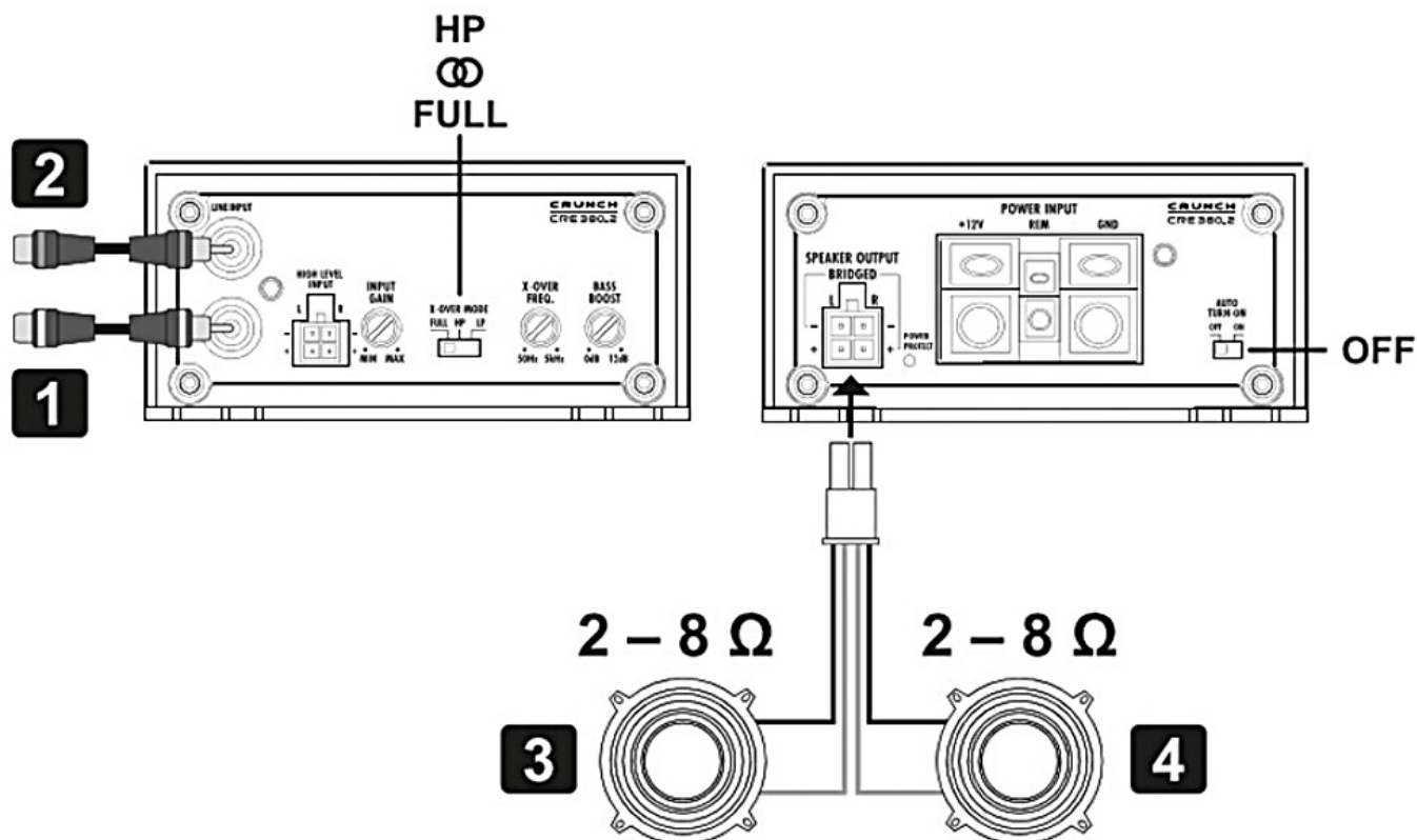
Rys. 3 — Praca 2-kanalowa (stereo). Jeden głośnik na każdy kanał; impedancja minimalna 2 Ω na kanał.
