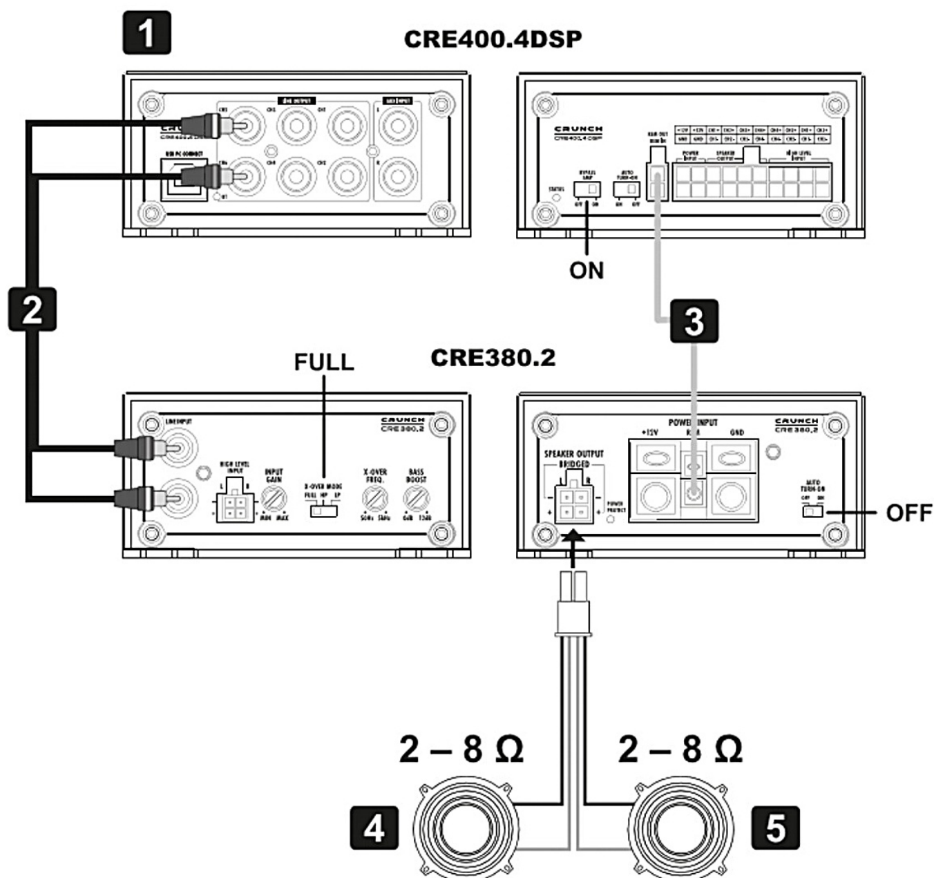
Rys. 5 — Praca 2-kanalowa z opcjonalnym procesorem dźwięku CRE400.4DSP, połączonym kablami RCA.
