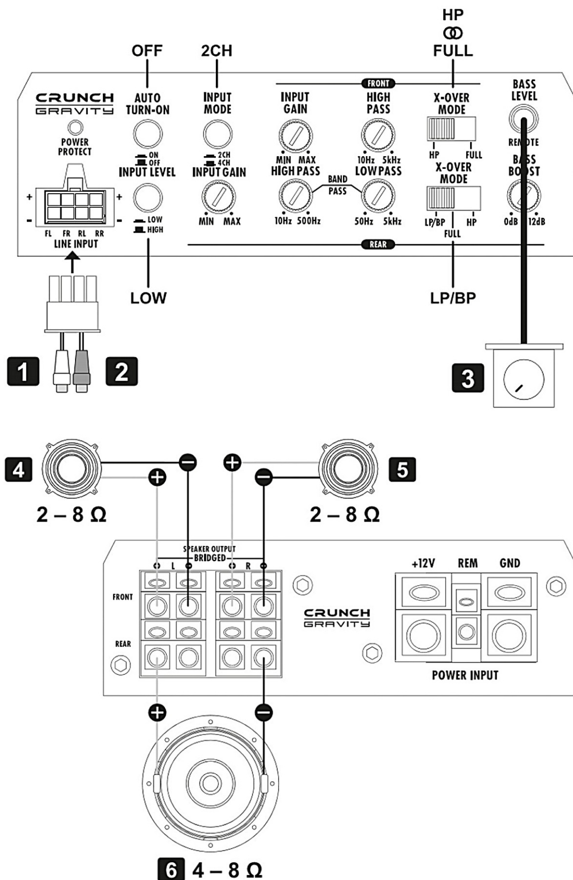
Rys. 4 — Praca 2 × stereo + 1 × mono. Para głośników FRONT oraz subwoofer na mostkowanej parze REAR (min. 4 \Omega ); X-OVER MODE > REAR w pozycji LP/BP, opcjonalnie zdalny regulator poziomu basów.
