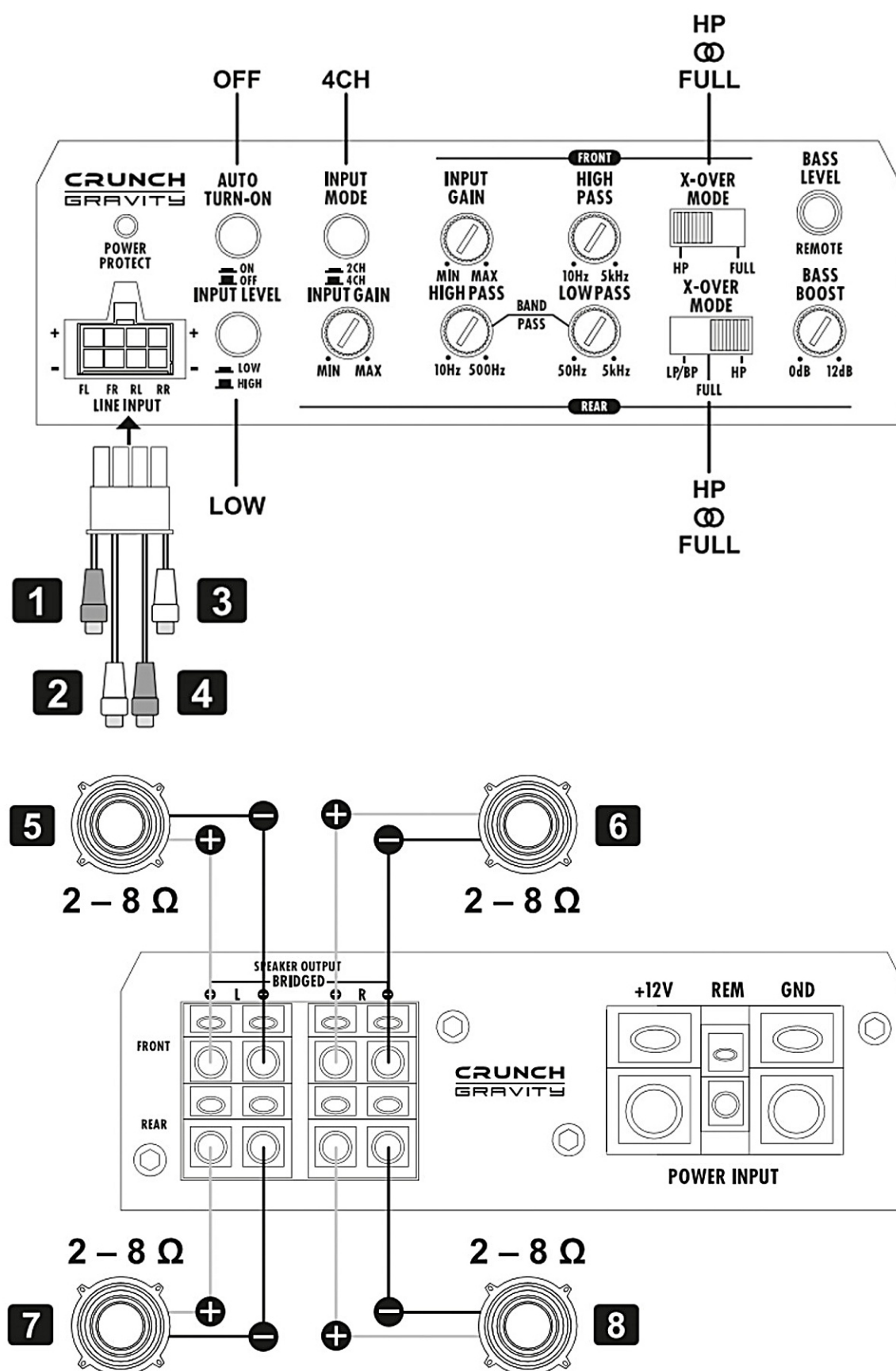
Rys. 3 — Praca 4-kanalowa (4 × stereo). Jeden głośnik na każdy kanał; impedancja minimalna 2 \Omega na kanał. Przełącznik INPUT MODE w pozycji 4CH, X-OVER MODE wg rodzaju głośników.
