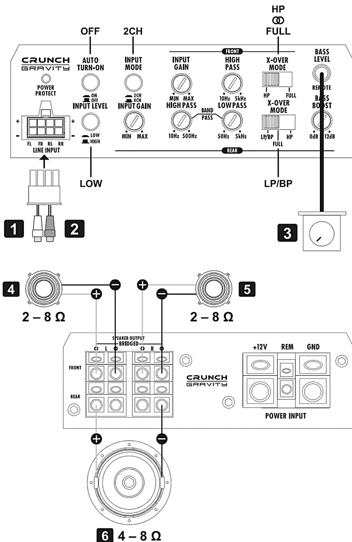
Rys. 4 — Praca 2 × stereo + 1 × mono. Para głośników FRONT oraz subwoofer na mostkowanej parze REAR (min. 4 Ω); X-OVER MODE > REAR w pozycji LP/BP, opcjonalnie zdalny regulator poziomu basów.
