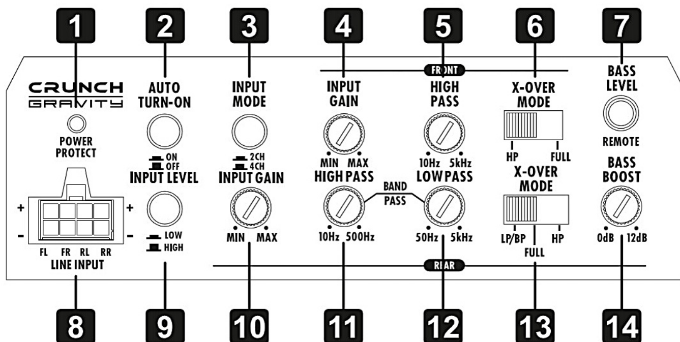
Rys. 1 — Przyłącza i elementy sterowania.
