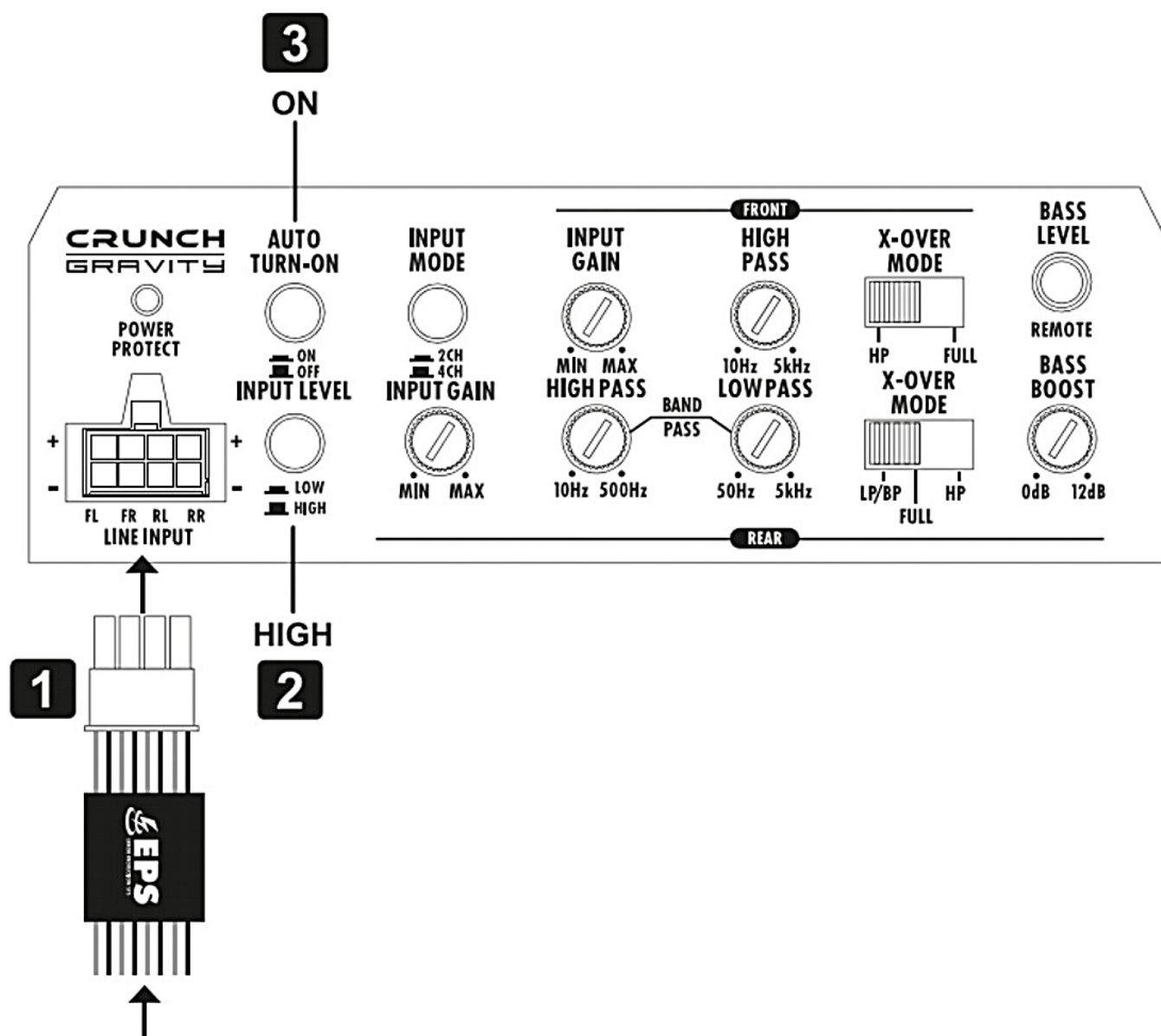
Rys. 5 — Wejścia wysokopoziomowe i automatyczne włączanie. Sygnał z kabli głośnikowych radia poprzez moduł EPS; przełącznik INPUT LEVEL w pozycji HIGH, AUTO TURN-ON w pozycji ON.
