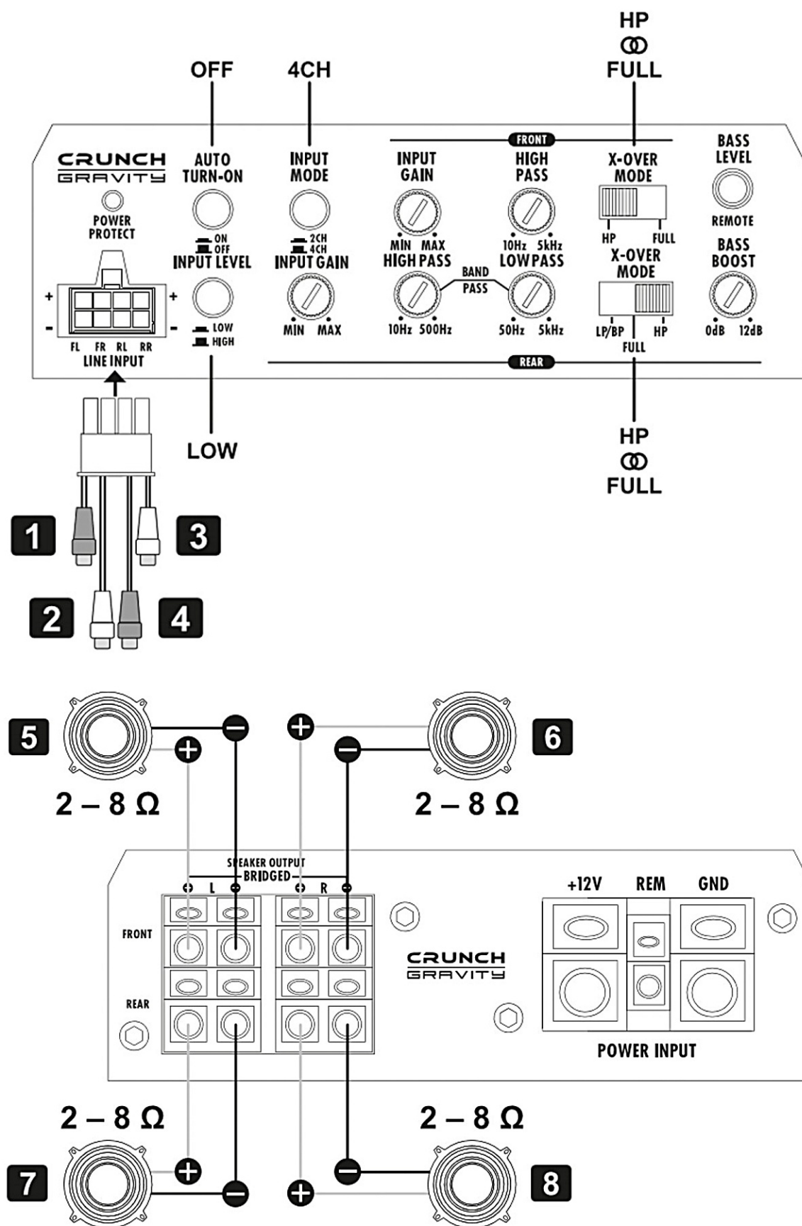
Rys. 3 — Praca 4-kanalowa (4 × stereo). Jeden głośnik na każdy kanał; impedancja minimalna 2 \Omega na kanał. Przełącznik INPUT MODE w pozycji 4CH, X-OVER MODE wg rodzaju głośników.
