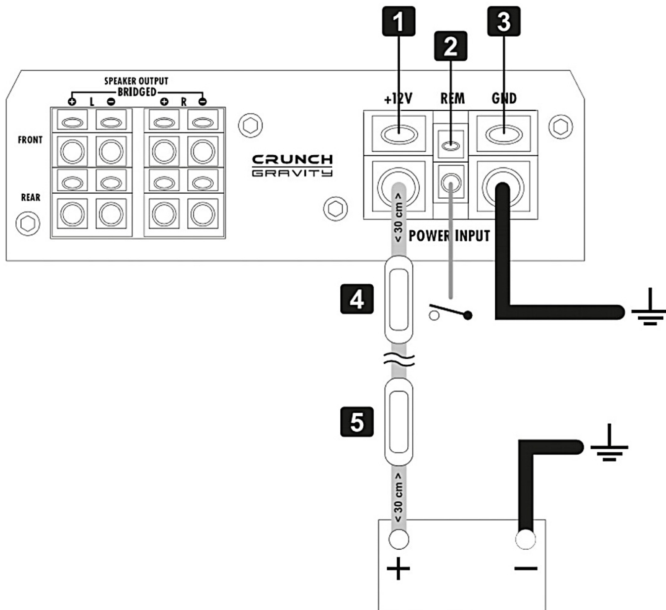
Rys. 2 — Podłączenie zasilania (1: +12V • 2: REM • 3: GND/masa • 4: zewnętrzny bezpiecznik dołączony do wzmacniacza • 5: dodatkowy bezpiecznik kabla +12V przy akumulatorze).
