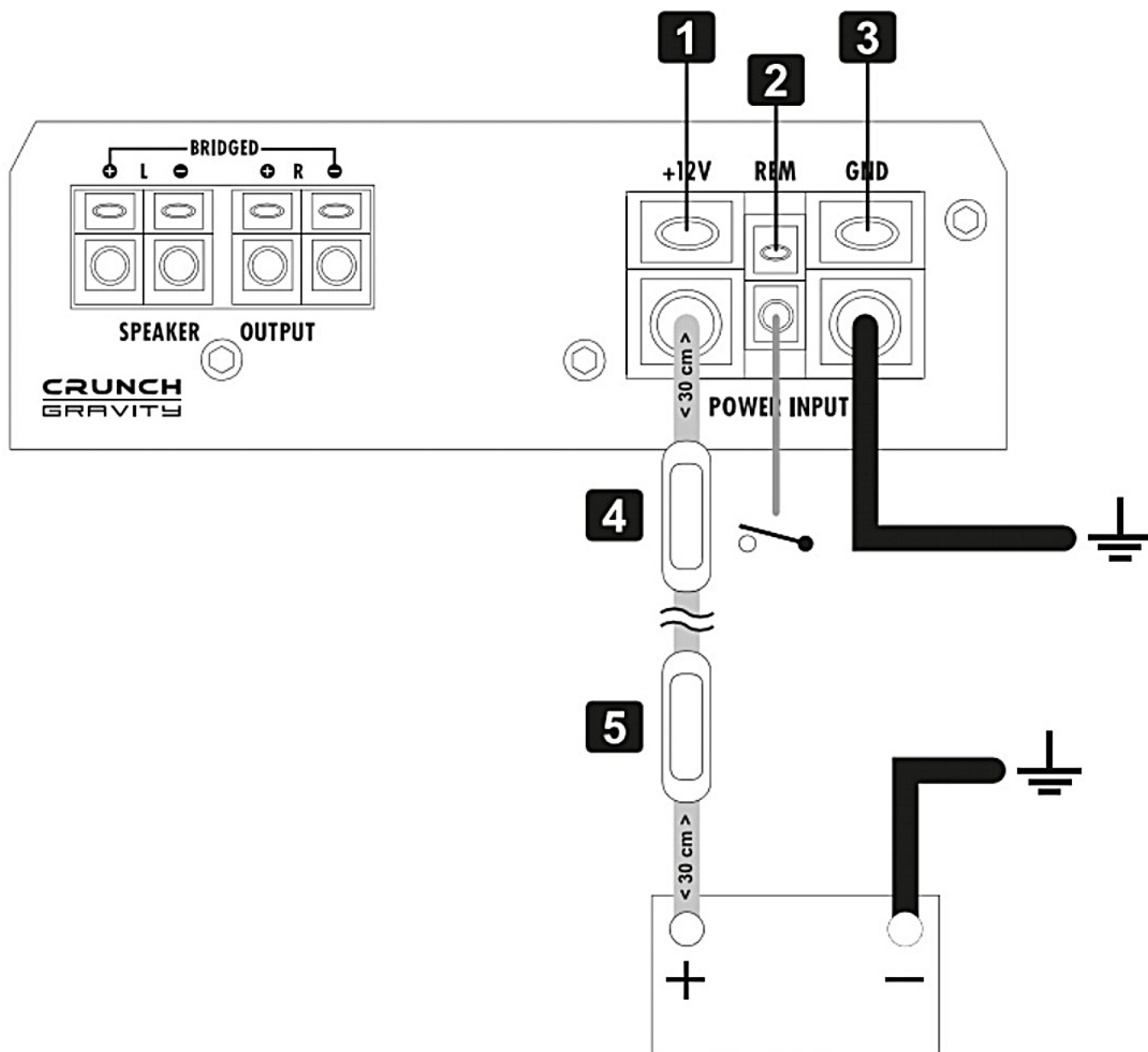
Rys. 2 — Podłączenie zasilania (1: +12V • 2: REM • 3: GND/masa • 4: dołączony bezpiecznik przy wzmacniaczu • 5: bezpiecznik przy akumulatorze)
