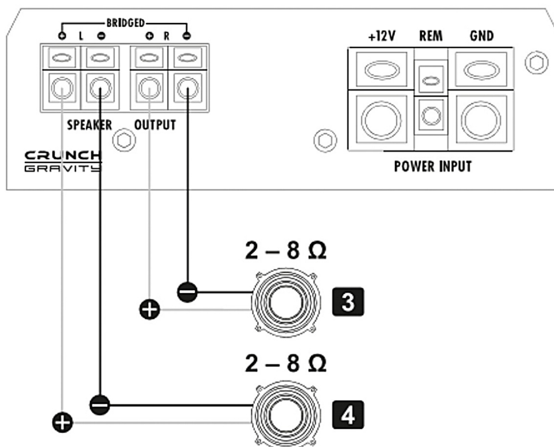
Rys. 3 — Praca 2-kanalowa. Sygnał L/R z radia przez RCA, po jednym głośniku na każdy kanał (impedancja 2 – 8 Ω); INPUT LEVEL w pozycji LOW, AUTO TURN-ON w pozycji OFF.
