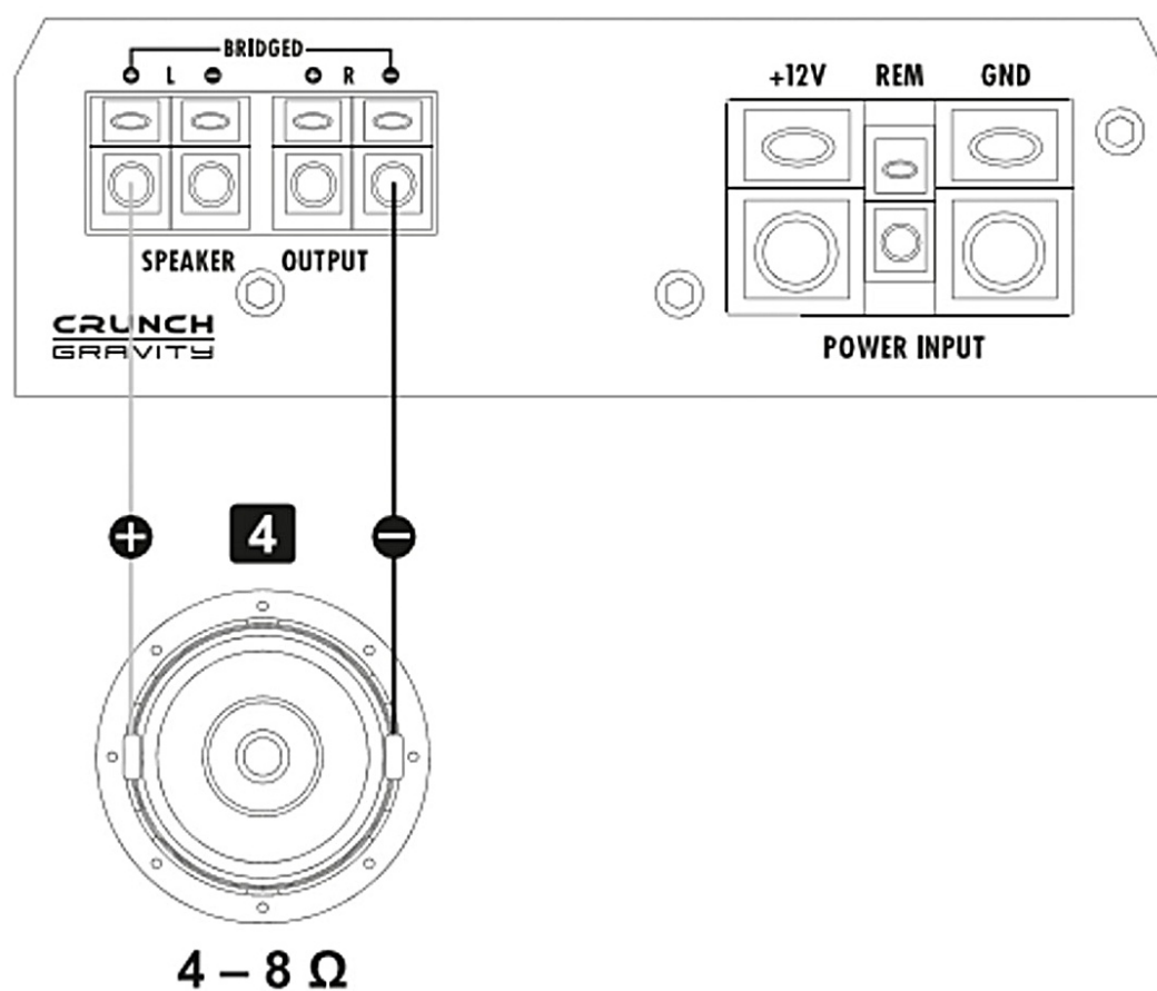
Rys. 4 — Praca mono mostkowa z subwooferem. Kanały połączone mostkowo (impedancja 4 – 8 \Omega ), pilot poziomu basów, X-OVER MODE w pozycji LP/BP.
