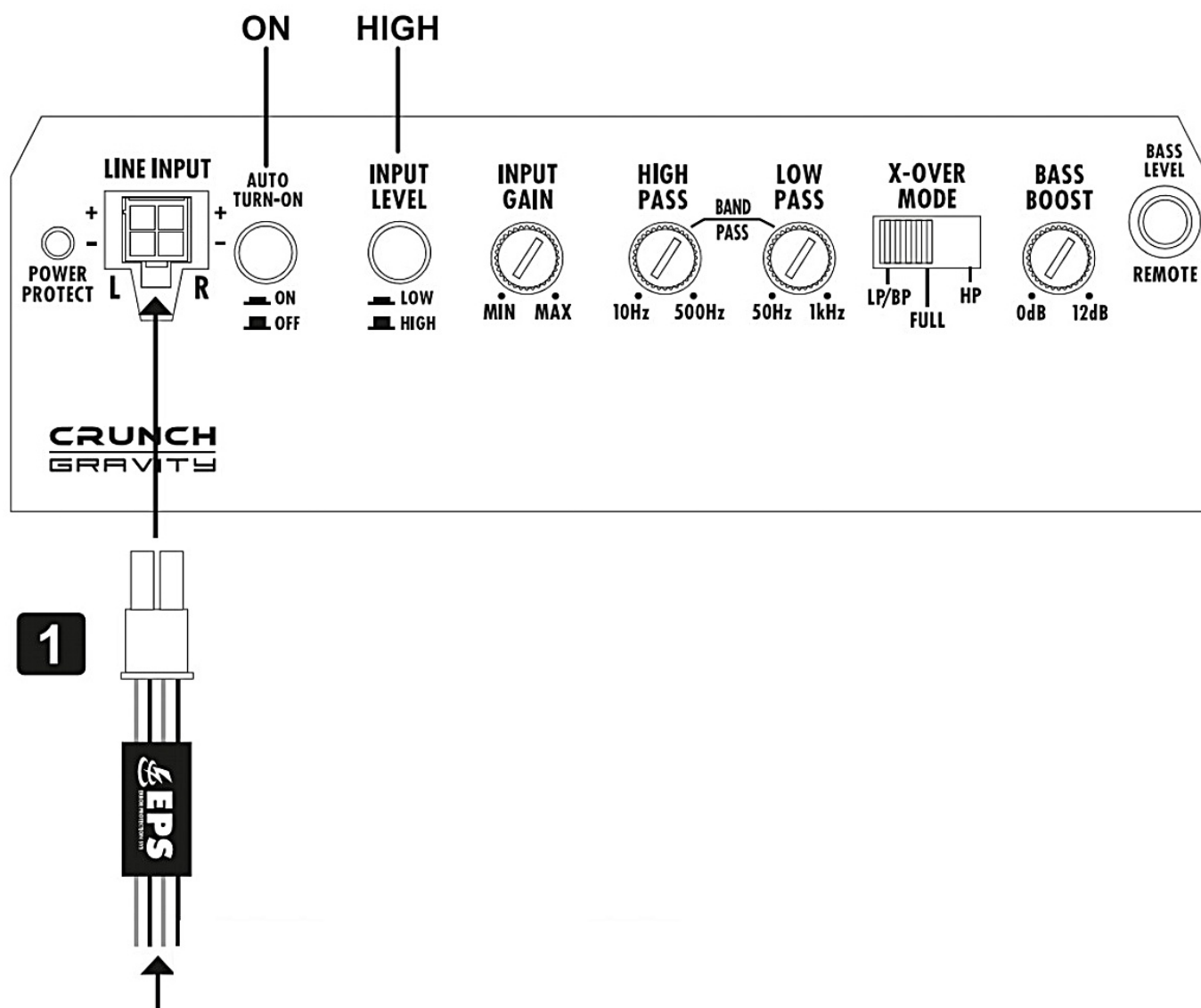
Rys. 5 — Wejścia wysokopoziomowe z modułem EPS. Sygnał z kabli głośnikowych radia; INPUT LEVEL w pozycji HIGH, AUTO TURN-ON w pozycji ON.
