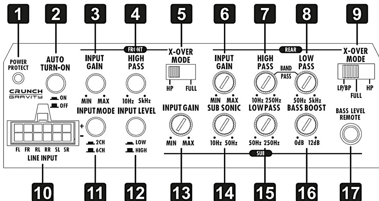
Rys. 1 — Przyłącza i elementy sterowania
