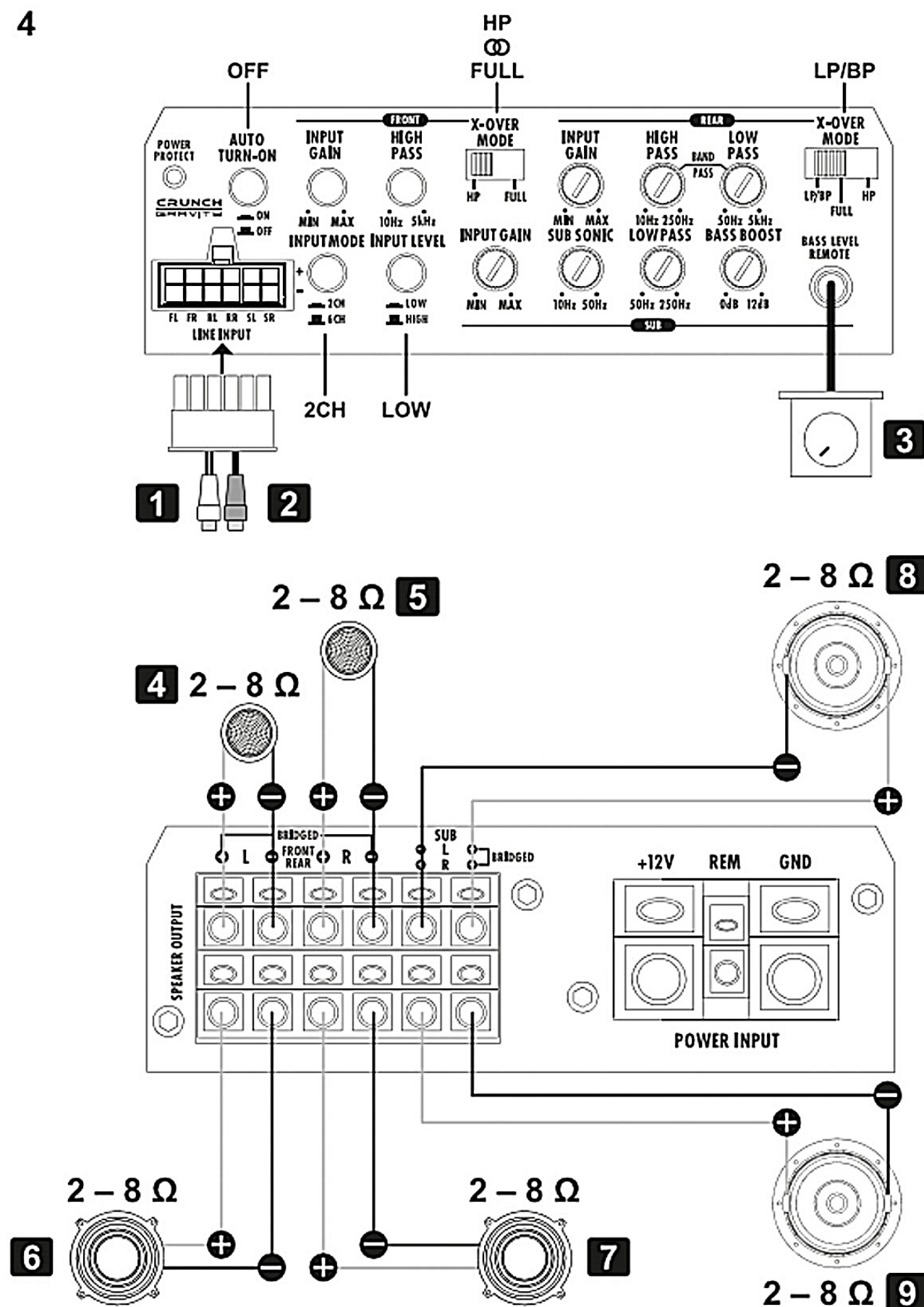
Rys. 4 — Układ aktywny zasilany z jednej pary wejść (tryb 2CH): głośniki wysokotonowe na kanałach FRONT (HP), głośniki nisko-/średnionowe na kanałach REAR (LP/BP) oraz subwoofery stereo na kanałach SUB.
