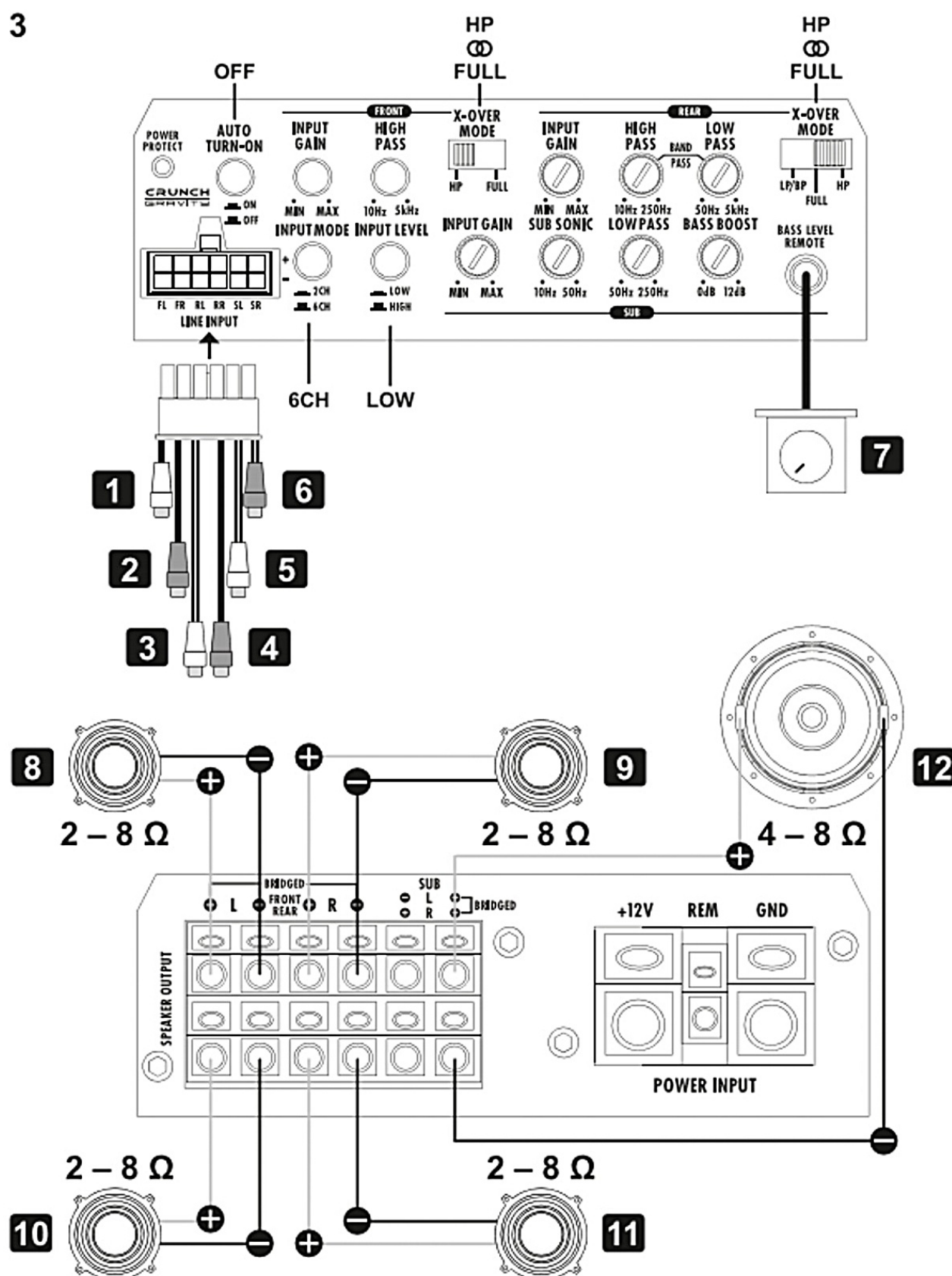
Rys. 3 — Praca 6-kanalowa. Cztery głośniki (front + tył) na kanałach FRONT i REAR oraz subwoofer na mostkowanych kanałach SUB. Wejścia w trybie 6CH, poziom LOW; impedancja minimalna 2 \Omega na kanał, 4 \Omega dla wyjścia mostkowanego.
