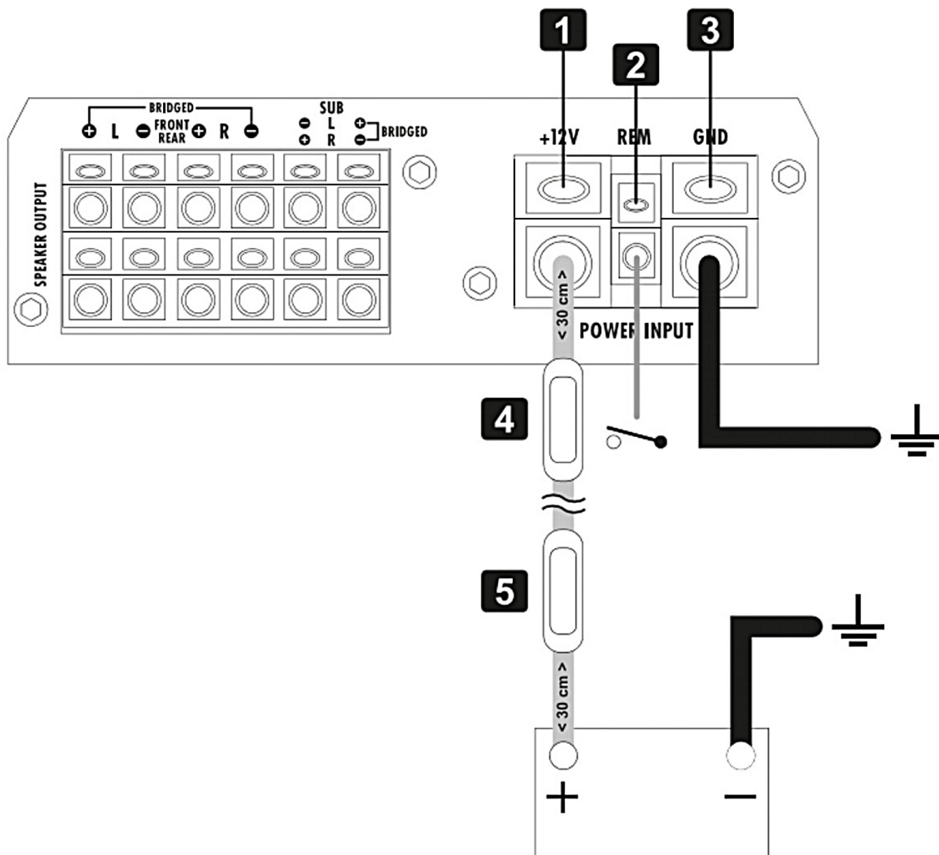
Rys. 2 — Podłączenie zasilania (1: +12V • 2: REM • 3: GND/masa • 4: bezpiecznik zewnętrzny dołączony • 5: dodatkowy bezpiecznik przy akumulatorze) oraz listwa wyjść głośnikowych (FRONT / REAR / SUB, z opcją mostkowania).
