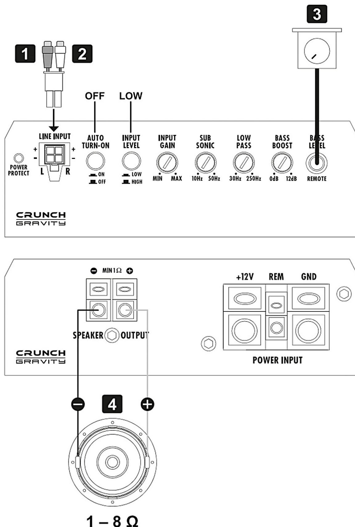
Rys. 3 — Praca monofoniczna. Sygnał z wyjść L/SUB i R/SUB radia (poz. 1 i 2) oraz pilot poziomu basów (poz. 3); subwoofer podłączony do wyjścia głośnikowego (poz. 4), impedancja minimalna 1 \Omega .
