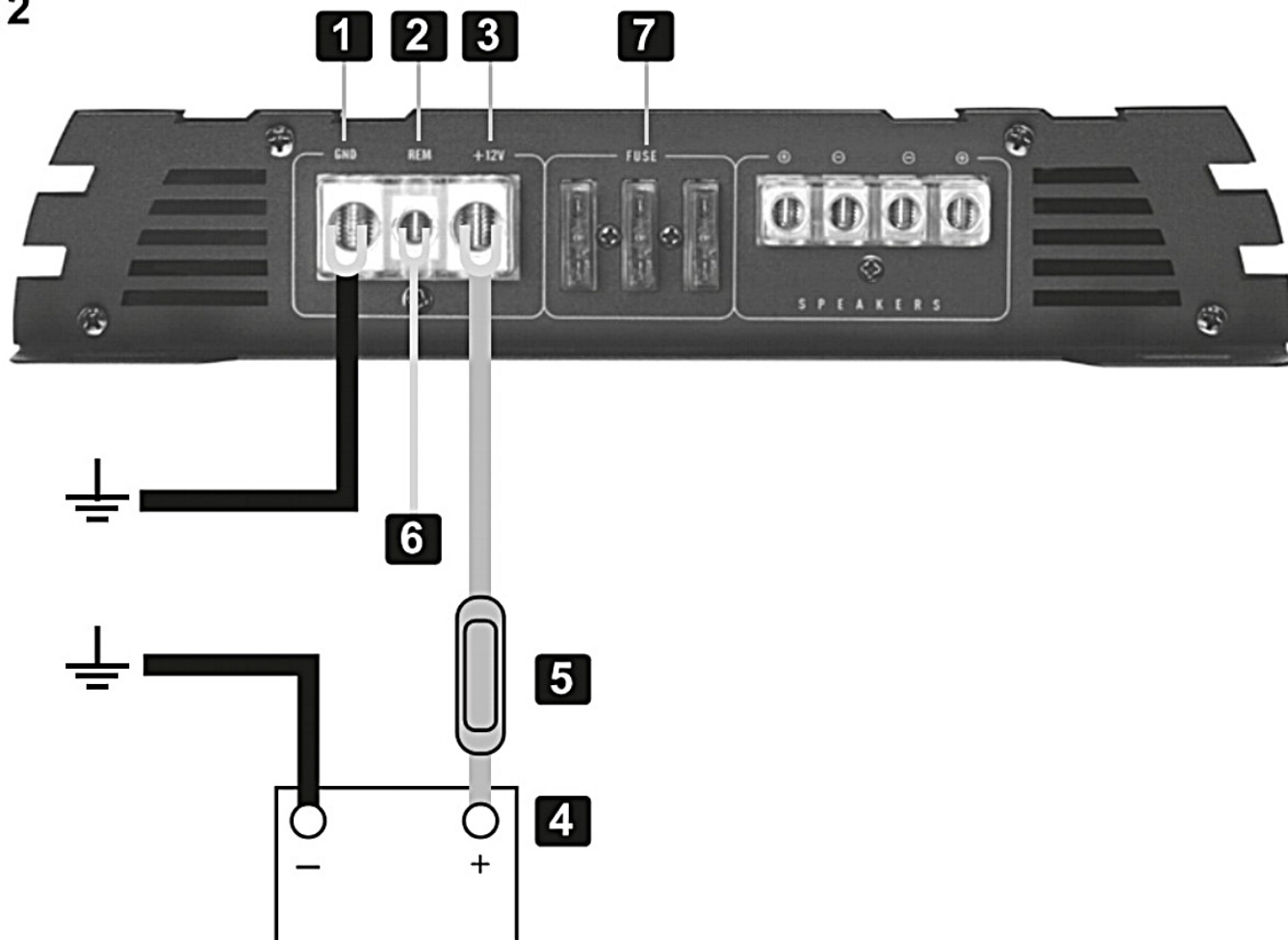
Rys. 2 — Podłączenie zasilania (1: GND/masa • 2: REM • 3: +12V • 4: akumulator pojazdu • 5: bezpiecznik liniowy przy akumulatorze • 6: przewód włączający z radia • 7: bezpieczniki wzmacniacza).
