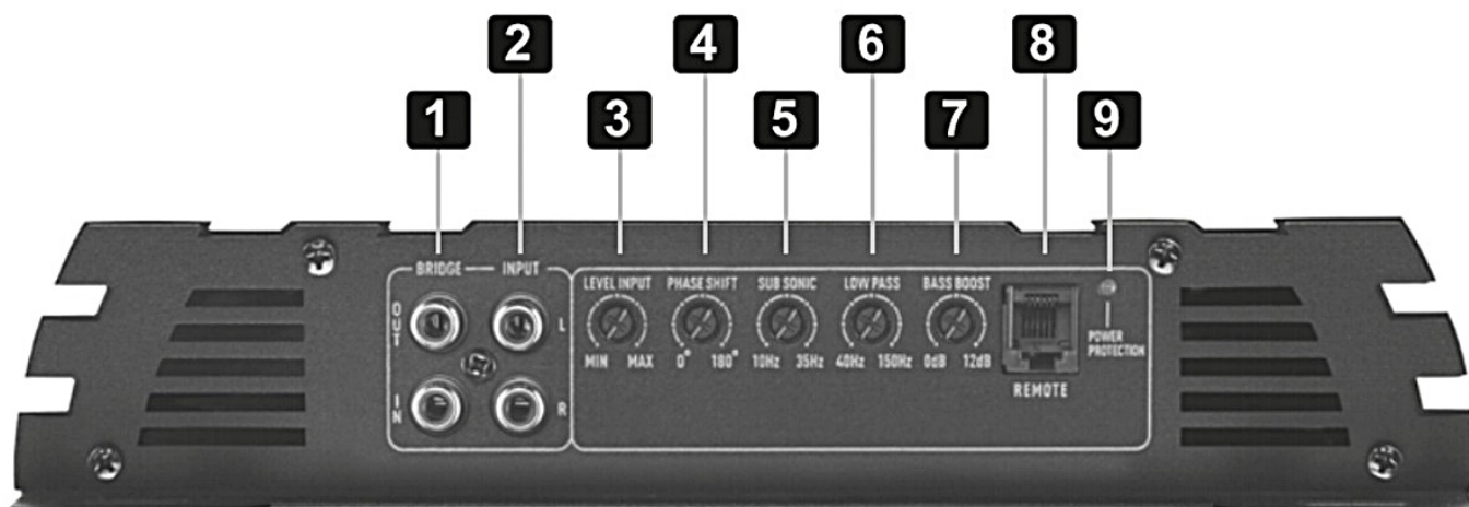
Rys. 1 — Przyłącza i elementy sterowania
