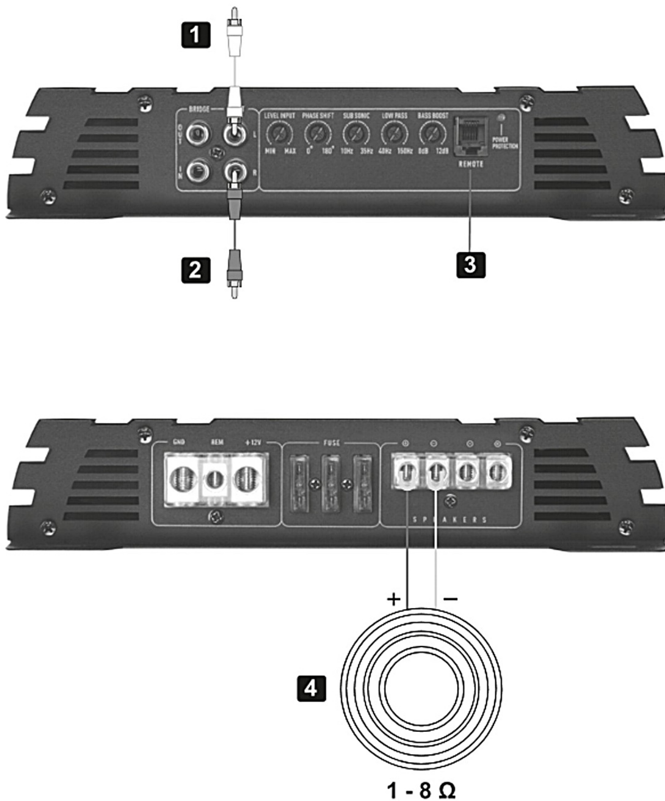
Rys. 3 — Praca monofoniczna z jednym subwooferem. Sygnał z wyjść radia (poz. 1 i 2), pilot poziomu basów (poz. 3), subwoofer (poz. 4) o impedancji minimalnej 1 Ω.
