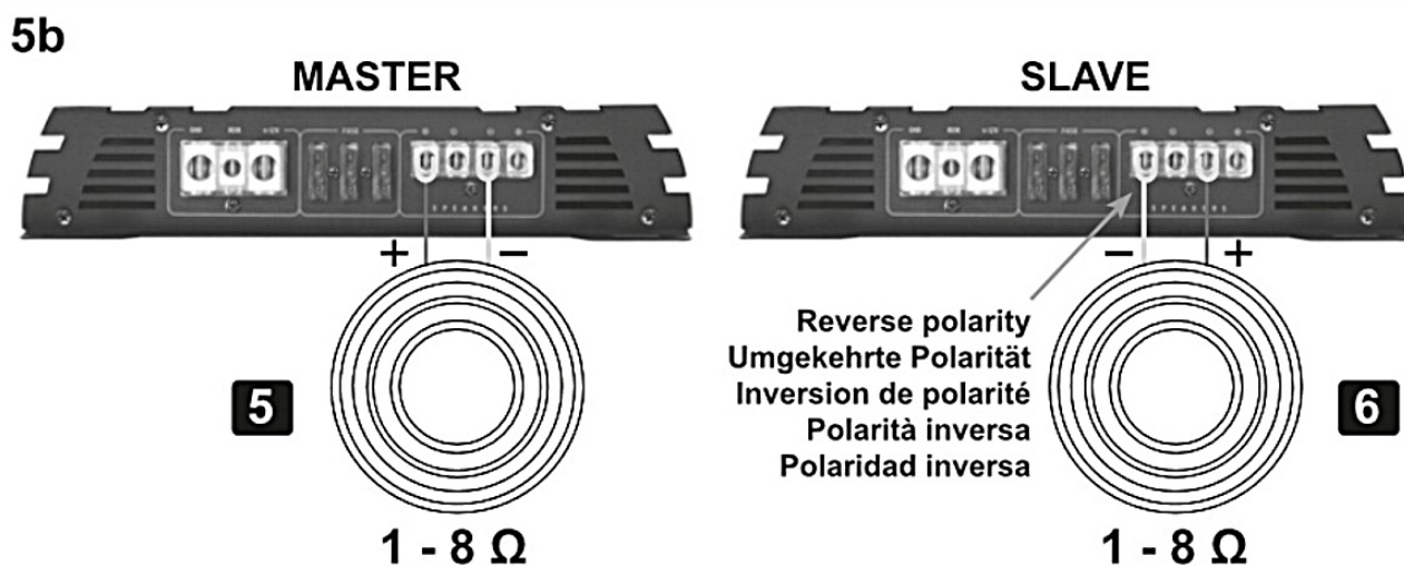
Rys. 5 — Tryb Master/Slave, osobne subwoofery. Połączenie RCA między Master a Slave (poz. 4); subwoofer wzmacniacza Master (poz. 5) i Slave (poz. 6) — każdy 1-8 Ω; subwoofer przy Slave podłączony z odwróconą polaryzacją (- do +).
