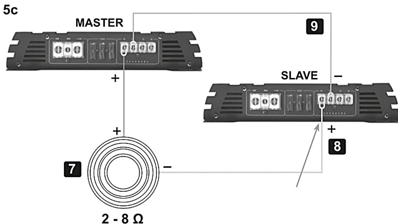
Rys. 5c — Tryb Master/Slave, jeden wspólny subwoofer (poz. 7), 2-8 Ω. Subwoofer podłączony przy wzmacniaczu Slave z odwróconą polaryzacją (poz. 8); zaciski ujemne (-) Master i Slave połączone razem (poz. 9).
