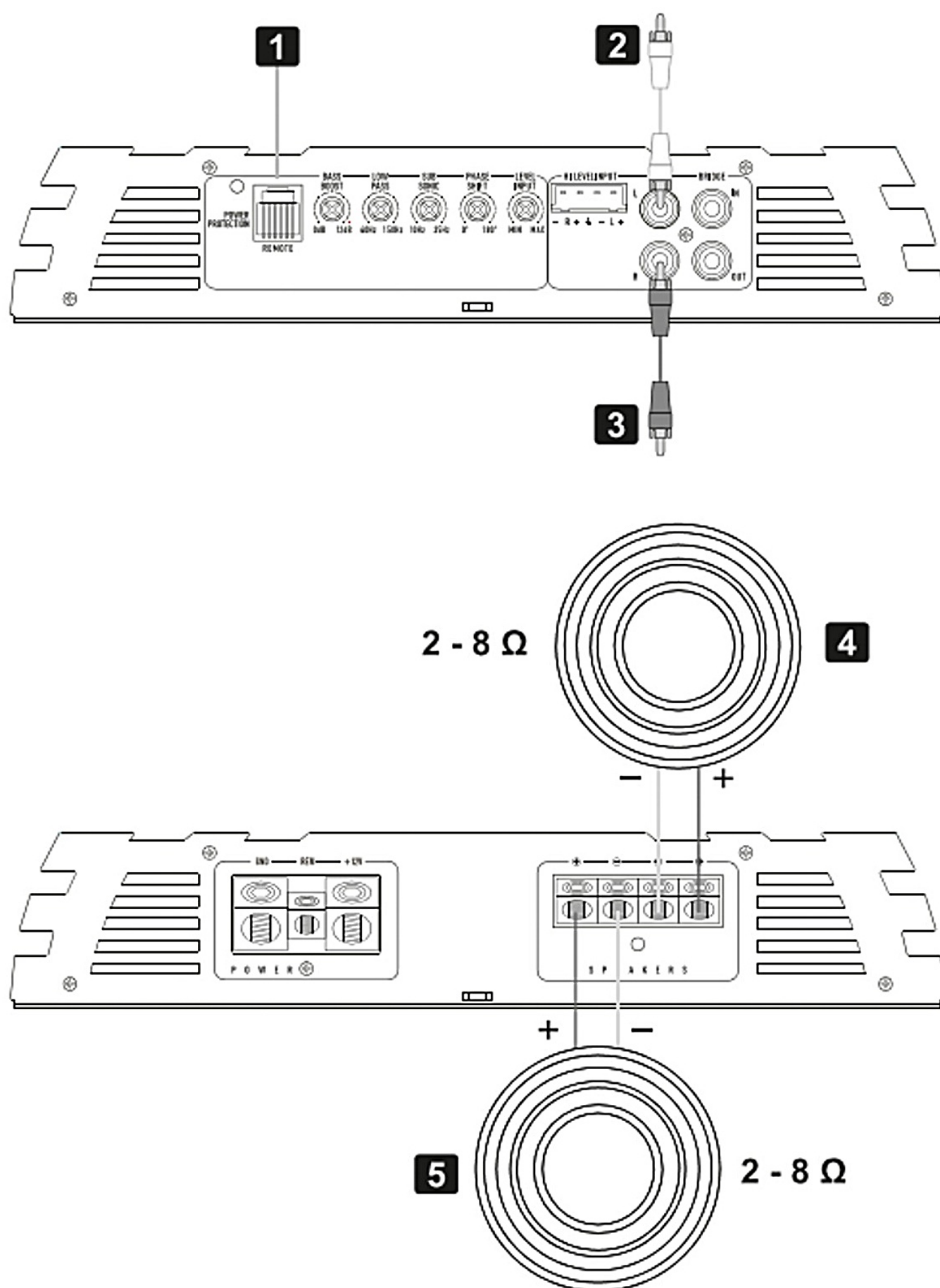
Rys. 4 — Praca monofoniczna z dwoma subwooferami. Sygnał z wyjść radia (poz. 2 i 3), pilot poziomu basów (poz. 1), dwa subwoofery (poz. 4 i 5), każdy o impedancji minimalnej 2 Ω.
