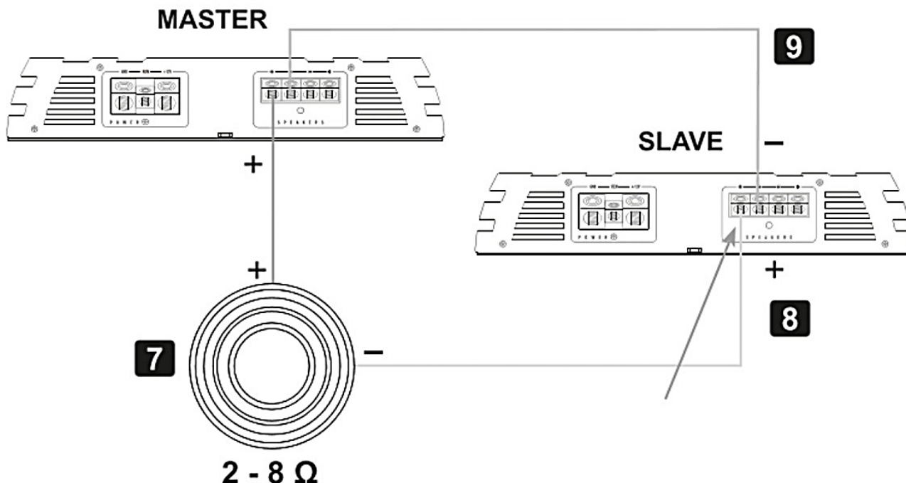
Rys. 5c — Tryb Master/Slave, JEDEN WSPÓLNY subwoofer (poz. 7), 2-8 Ω. UWAGA: subwoofer podłączyć przy wzmacniaczu Slave z ODWRÓCONĄ POLARYZACJĄ — minus (-) wzmacniacza do plusa (+) głośnika (poz. 8). Dodatkowo zaciski ujemne (-) wyjść głośnikowych Master i Slave połączyć ze sobą (poz. 9).
