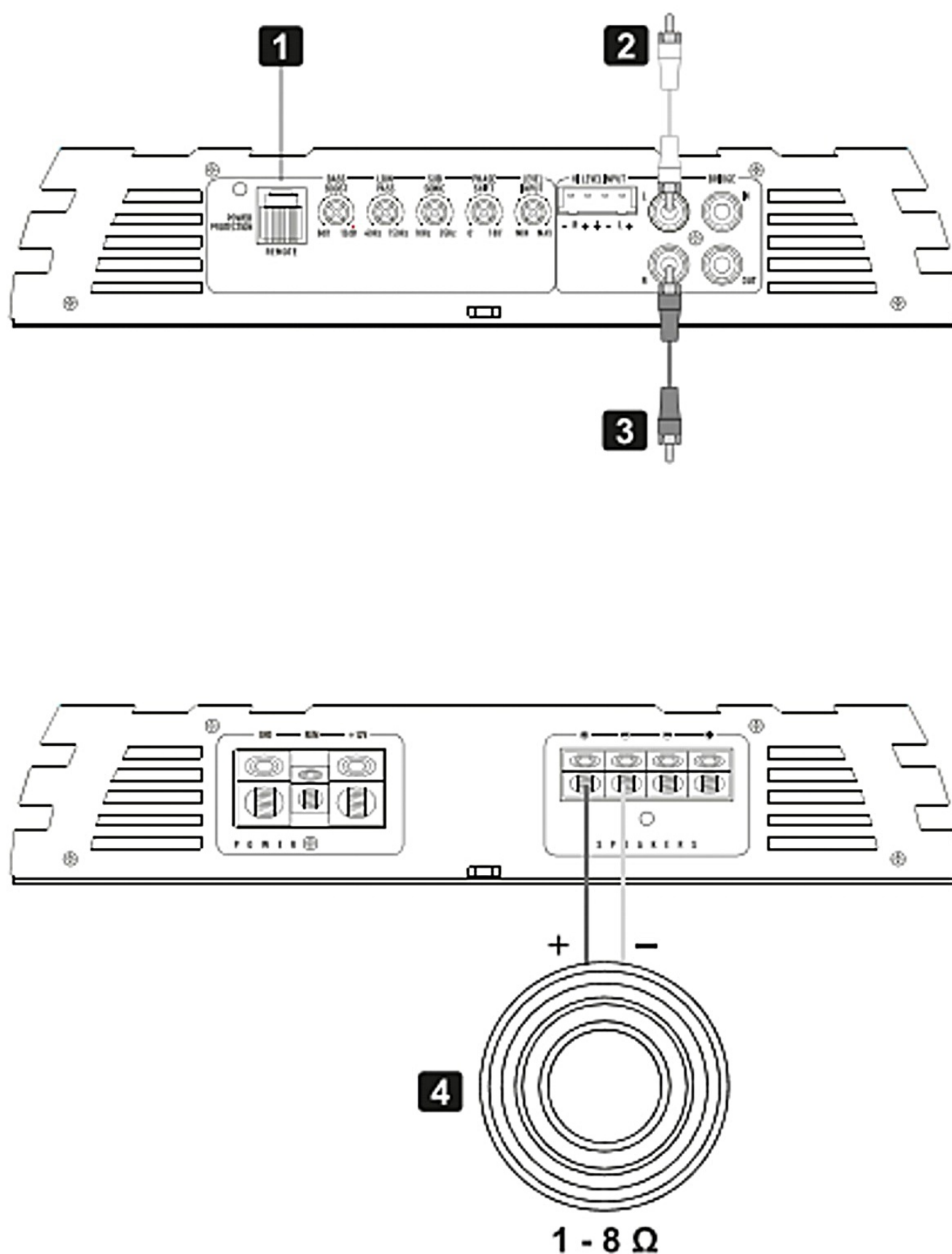
Rys. 3 — Praca monofoniczna z jednym subwooferem. Sygnał z wyjść radia (poz. 2 i 3), pilot poziomu basów (poz. 1), subwoofer (poz. 4) o impedancji minimalnej 1 Ω.
