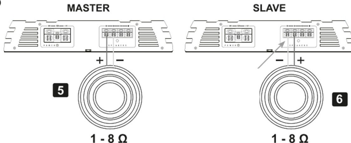
Rys. 5 — Tryb Master/Slave, OSOBNIE subwoofery. Sygnał z radia (poz. 2 i 3) do wzmacniacza Master, pilot poziomu basów (poz. 1), połączenie RCA z OUT MASTER do IN SLAVE (poz. 4). Subwoofer Master (poz. 5) i Slave (poz. 6) — każdy 1-8 Ω. UWAGA: subwoofer przy wzmacniaczu Slave podłączyć z ODWRÓCONĄ POLARYZACJĄ — minus (-) wzmacniacza do plusa (+) głośnika i odwrotnie.
