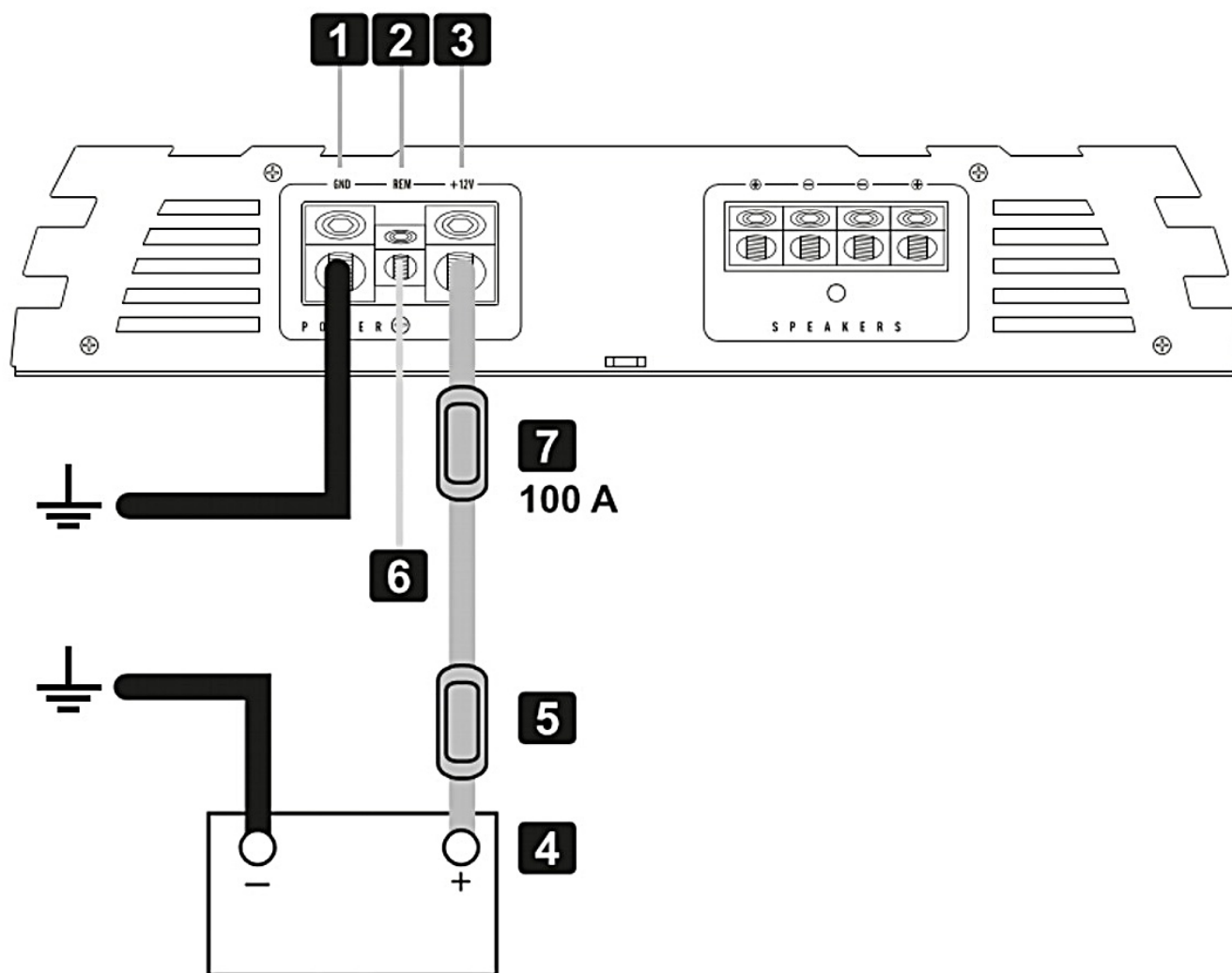
Rys. 2 — Podłączenie zasilania (1: GND/masa • 2: REM • 3: +12V • 4: akumulator pojazdu • 5: bezpiecznik liniowy przy akumulatorze • 6: przewód włączający z radia • 7: dołączony bezpiecznik liniowy 200 A przy wzmacniaczu).
