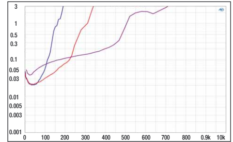
Die VX5000 PRO produziert nur an 1 Ohm minimal erhöhtes Klirren. Bei der 1 % Marke macht sie ihre 5 Kilowatt, lässt man 2 % zu, sind es 6,5 Kilowatt
